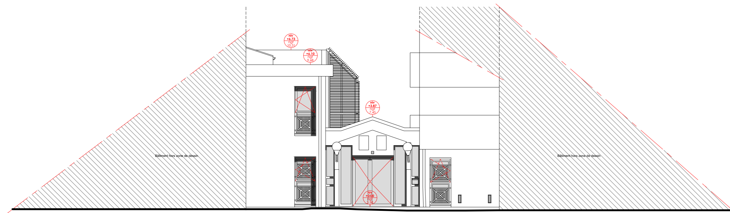
Façade Sud
