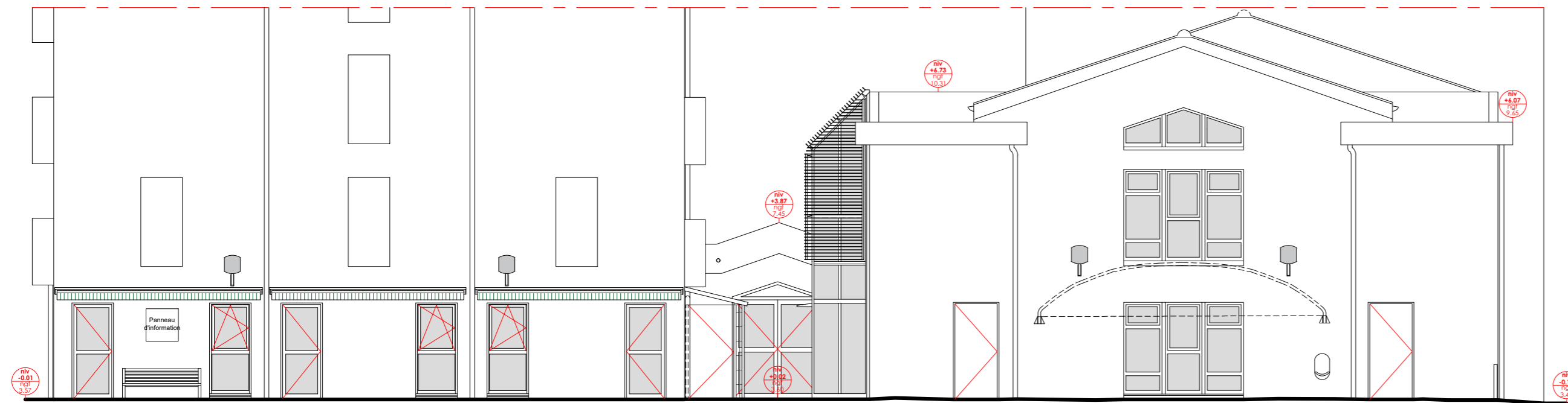
Façade Nord
